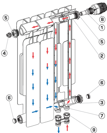
Рис. 1. Устройство радиатора
